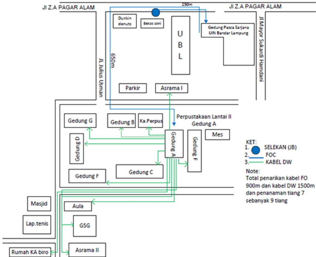
Gambar C.2 Infrastruktur network fiber optic (FO) di lingkungan pascasarjana UINRIL hingga tahun 2023
